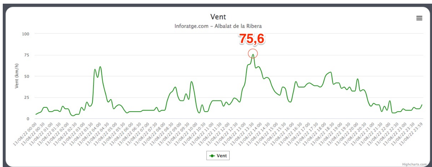
Ráfagas de viento registradas en ALBALAT DE LA RIBERA el 13/08/22 https://inforatge.com/meteo-albalatdelaribera
